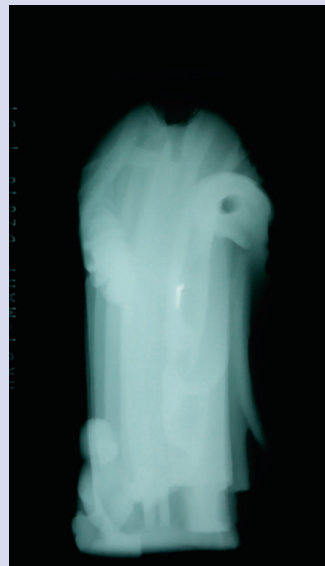
Figur D in der Röntgenaufnahme: Bei der hohen energetischen Strahlung, die benötigt wird, um den Sandstein zu durchdringen, wird der hölzerne Kopf völlig durchstrahlt und ist deshalb nicht sichtbar. © Butz, 2018
