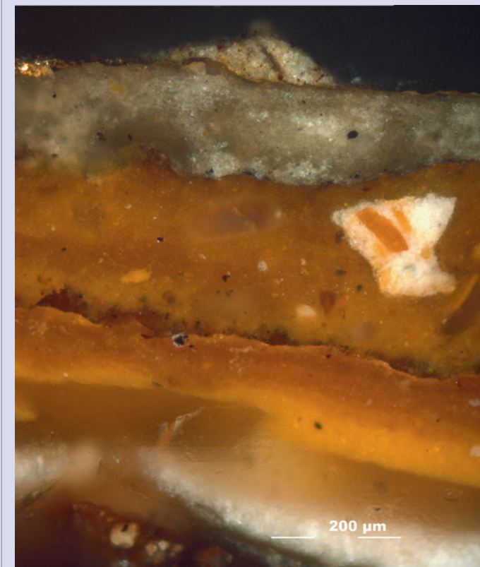
Anschliff der Probe D2 (Vergoldungen) unter 200-facher Sehfeldvergrößerung, Hellfeld, gekreuzte Polarisatoren. In der unteren Bildhälfte erkennt man die mehrschichtige Polimentvergoldung (Goldblatt horizontal in der Bildmitte). Darüber befindet sich eine Schicht grobkörnigen Poliments. © Butz, 2018
